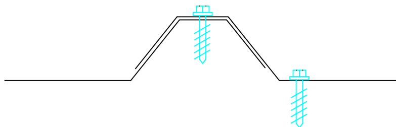
R Panel edge lap
